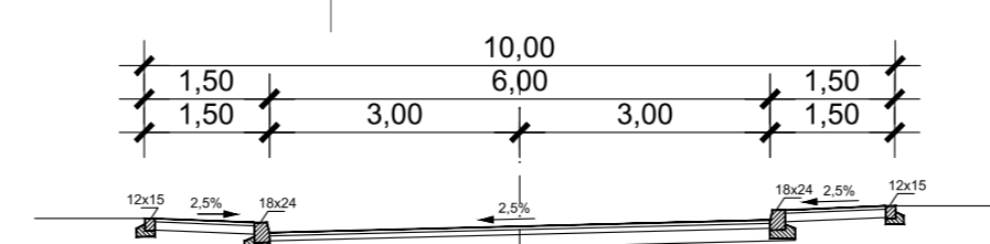
NORMALNI POPREČNI PROFIL mj. 1:100
